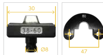
各押ダイス
