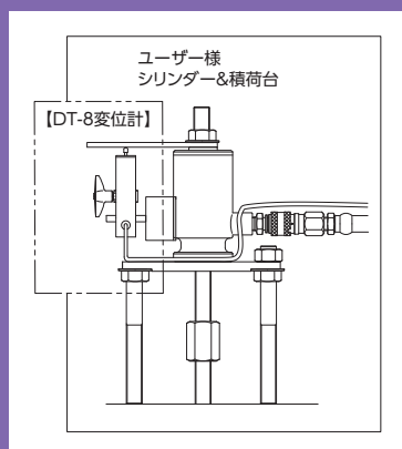
システム図
