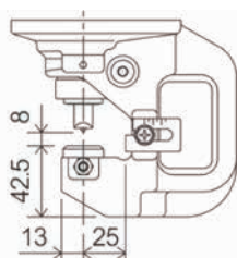
ヘッド部基本寸法 (mm)
