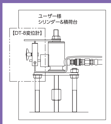
システム図
