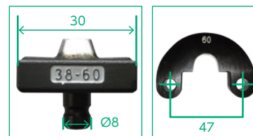
EV-60DL・S-60ES用各押ダイス 受けダイス
