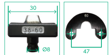
EV-60DL・S-60ES用各押ダイス 受けダイス
