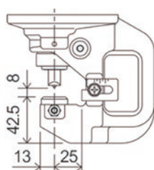
ヘッド部基本寸法 (mm)
